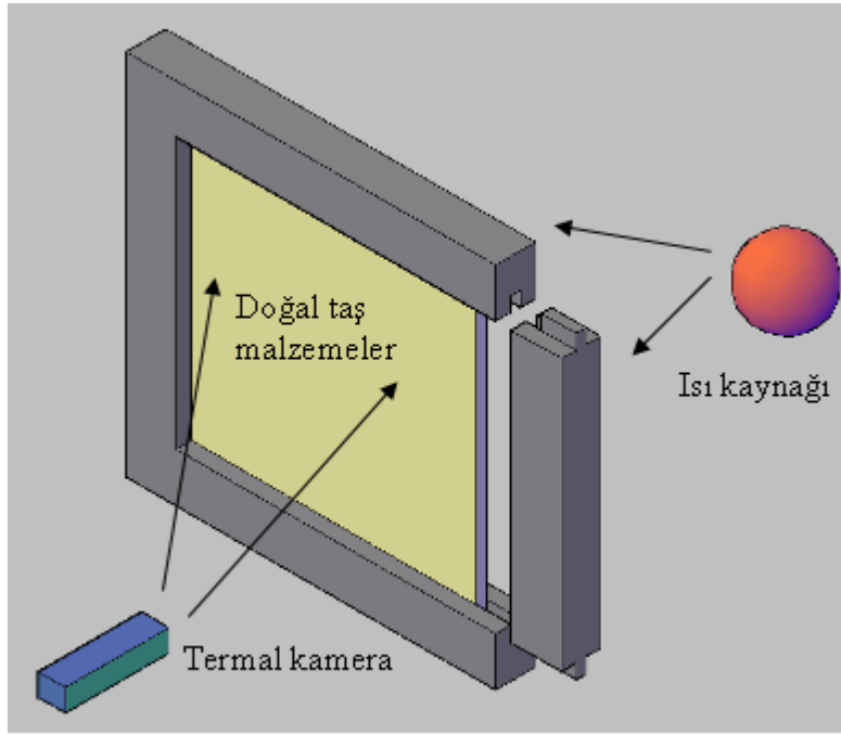
Şekil 5. Deneysel çalışma modeli
