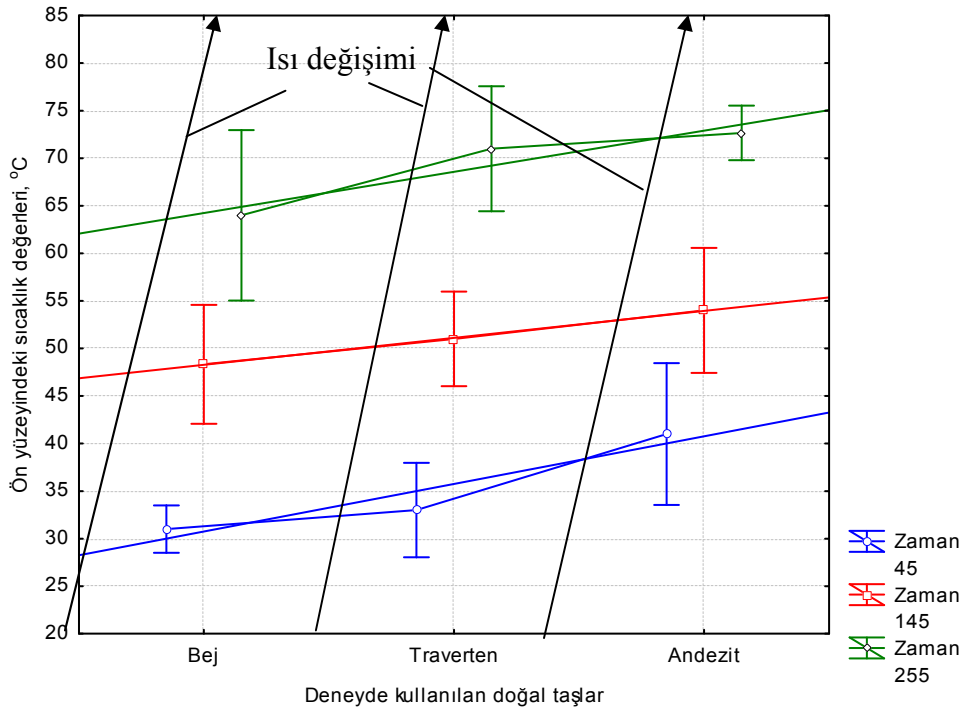
Şekil 6. Doğal taşlara göre zaman*sıcaklık değişimi
